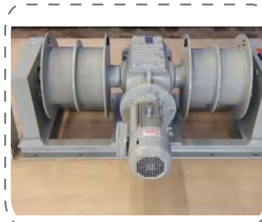
Treuil à tambours multiples
