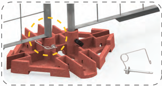
Goupille Standard
